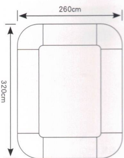
組合示意圖1
