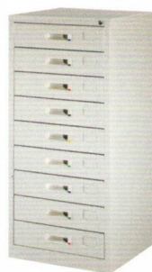
25012 單九層 W46xD45xH106(cm)
