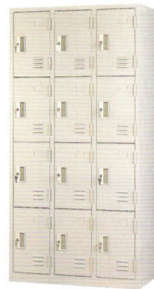
25006 12人衣櫥 W88xD51xH178(cm)
