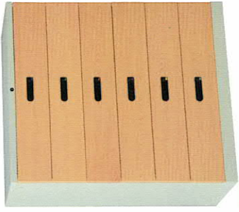
附加採購 02308 六層式小抽屜鋼製公文櫃 W900xD450xH1062(mm)
